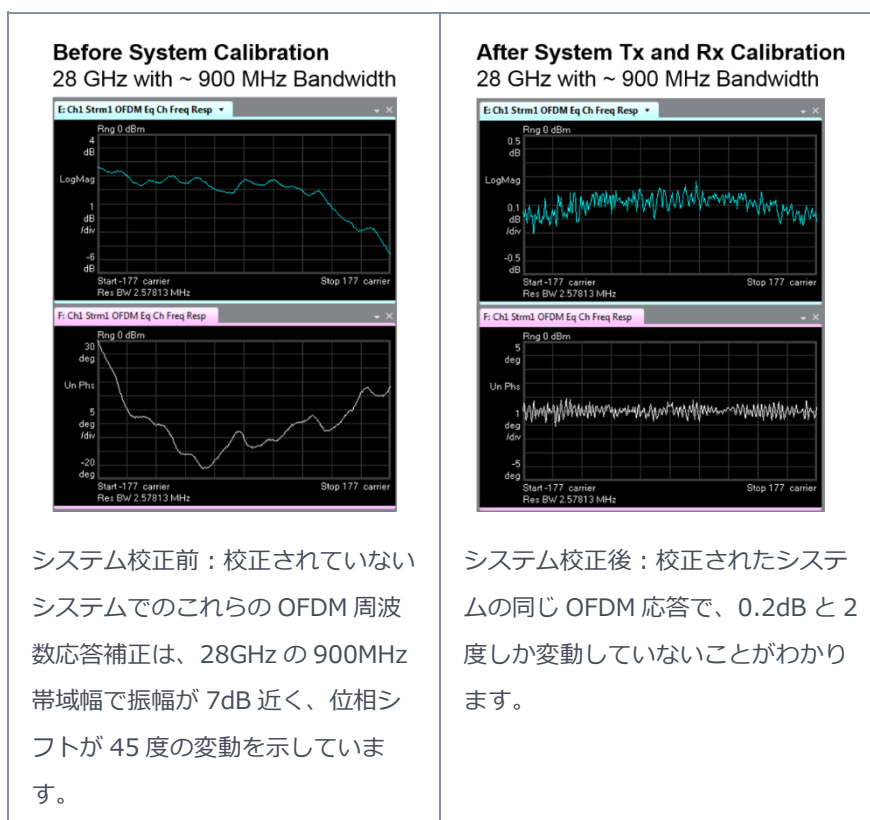
図5：校正前後の OFDM 変調周波数特性
