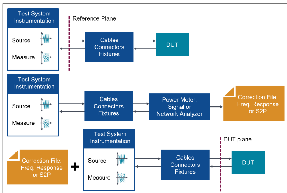
図 2：RF 校正のセットアップ
