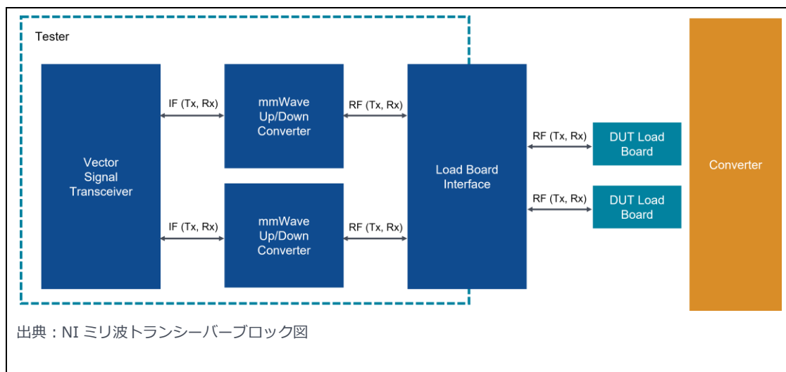
図 1：ミリ波 RF テストのための検査システム構成
