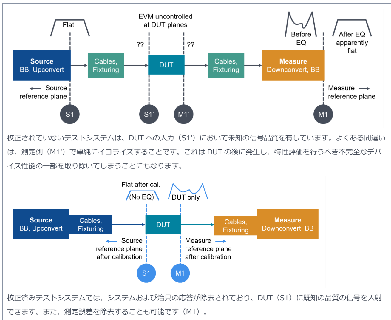
図 4：校正による DUT へのテストプレーンの移動
