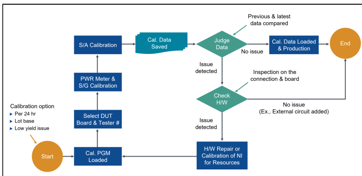
図 3：スカラー RF の校正手順
