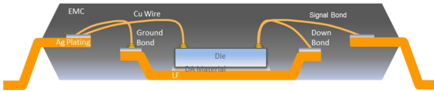
图 2: ExposedPad TQFP 横截面。
