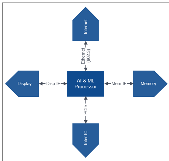
图 4：典型 (AI) 处理器及其数字高速测试接口。
