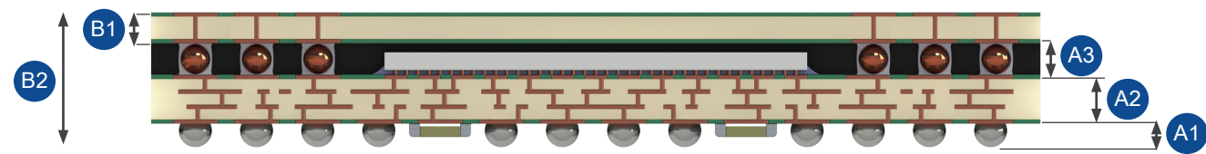
介质层 PoP 堆叠规格表 ( 参考范例 )
