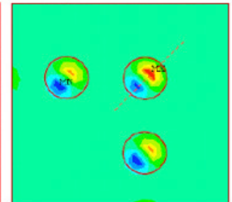
Die corner에 칩 어태치 후 Low-k 층의 최대 인장 응력 시뮬레이션
