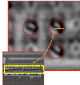
SAT에 의한 화이트 범프 칩 코너의 Low-k 층 데미지
