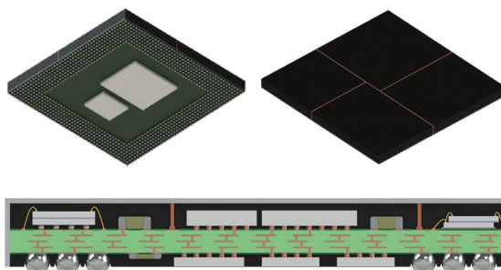
上面/底面組立、モールドイング、コンフォーマル/およびコンパートメントシールド
